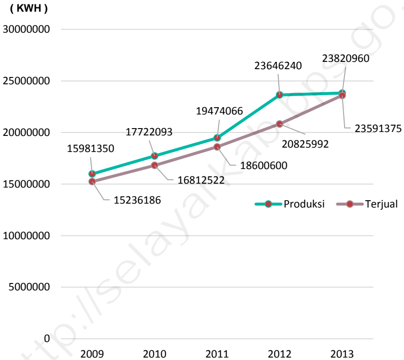
GRAFIK/Graph 6.2. JUMLAH LISTRIK PLN YANG DIPRODUKSI DAN TERJUAL DI KABUPATEN KEPULAUAN SELAYAR TAHUN 2009-2013 Number of Electrical Production and Sold in Kepulauan Selayar Regency Year 2009 - 2013
